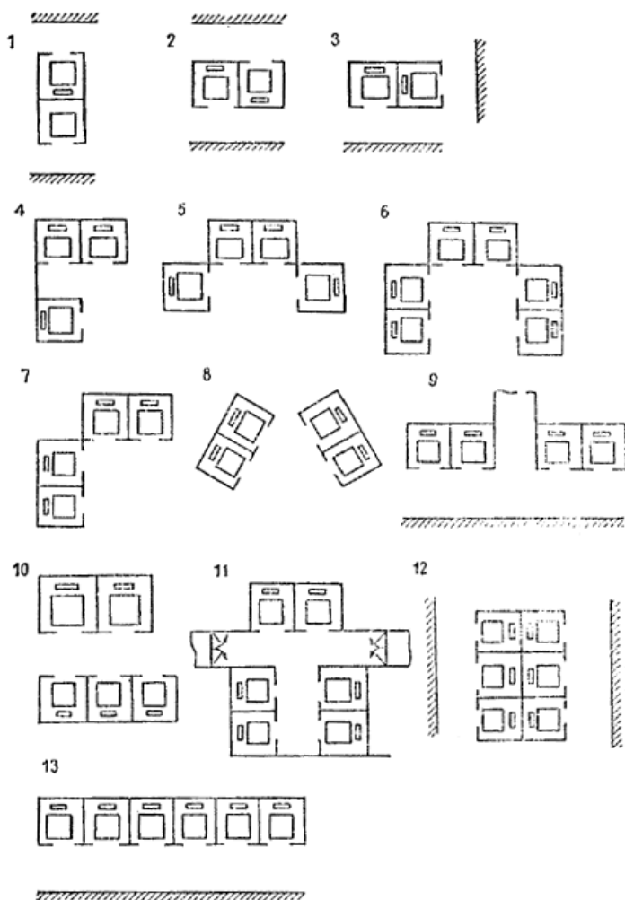
Рис. 9. Примеры схем нерекондуемого расположения лифтов
