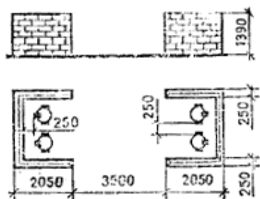
Рис. 18. Схема площадки под мусоросборники вместимостью 0,1 м 3
