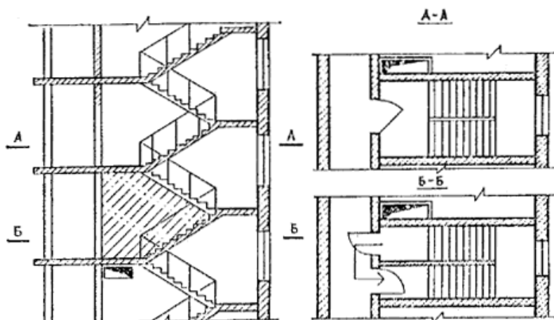
Рис. 25. Устройство рассечки между этажами в лестничной клетке с подпором воздуха
