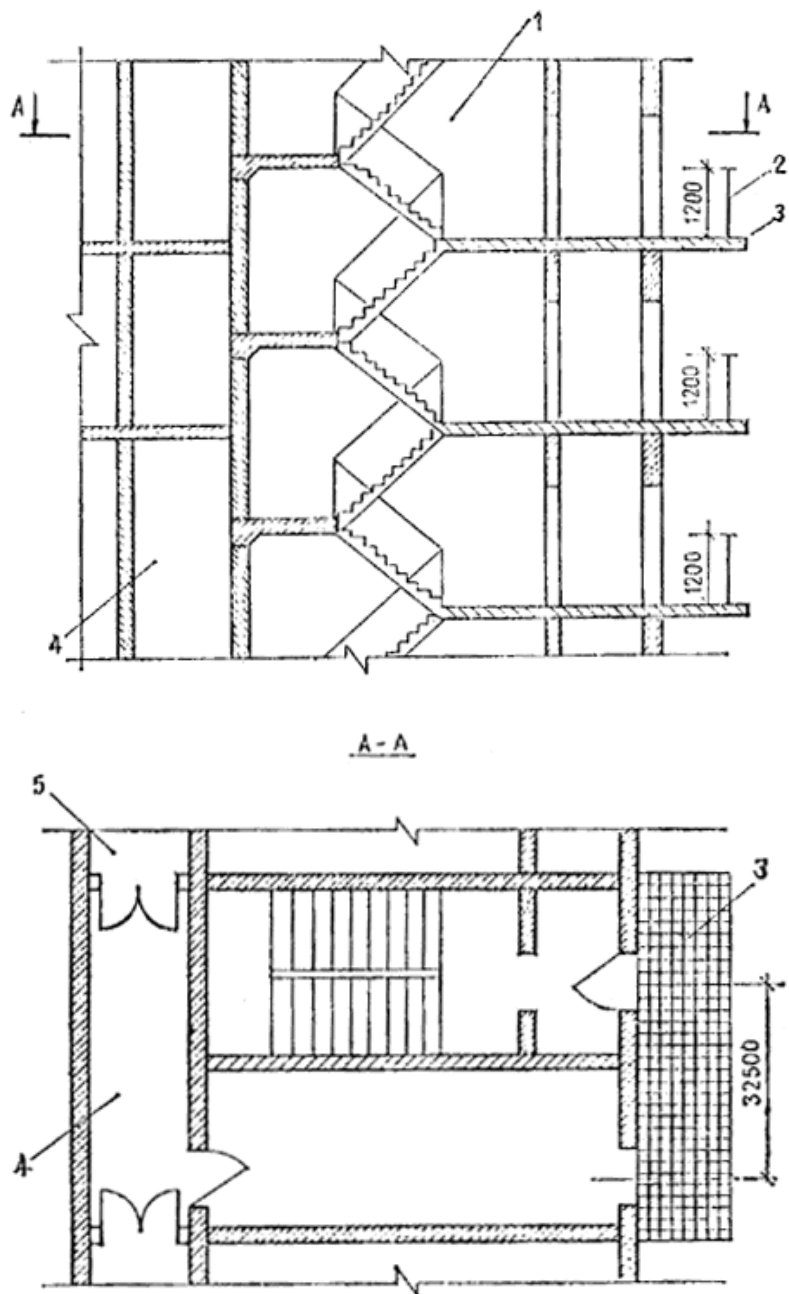
Рис. 24. Пример планировочного решения лестничной клетки с переходом через наружную воздушную зону по балконам
