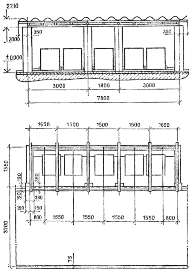
Рис. 20. Площадка крытая для пяти контейнеров
