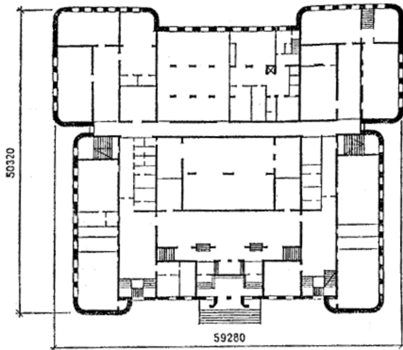
Рис. 2. Компактное решение здания (на примере общеобразовательной школы) с одним входом и двойным тамбуром, обеспечивающим изменение направления движения
