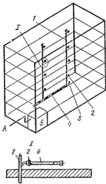
Рис. 10. Схема вакуумной комбинированной пылеуборки
