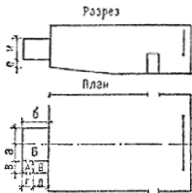
Рис. 6. Схема планировки кинопроекционного комплекса конференц-зала
