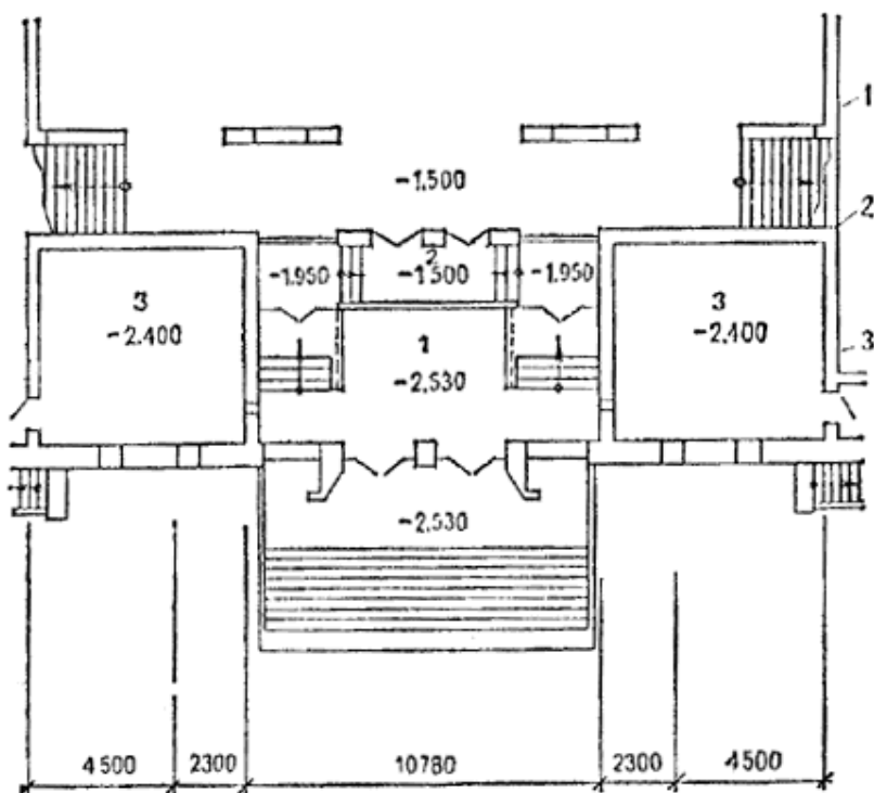
Рис. 3. Фрагмент (вход в здание)
