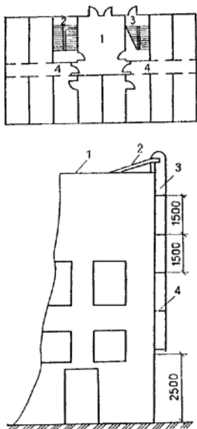
Рис. 21. Пример планировочного решения по устройству выходов из лестничных клеток через один вестибюль
