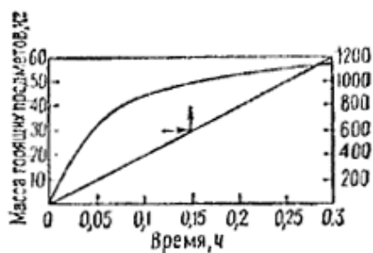
Рис. 23. Зависимость продолжительности начальной стадии пожара от площади пола и максимальной по времени среднеобъемной температуры от массы горящего вещества на 1 \text{ м}^2
