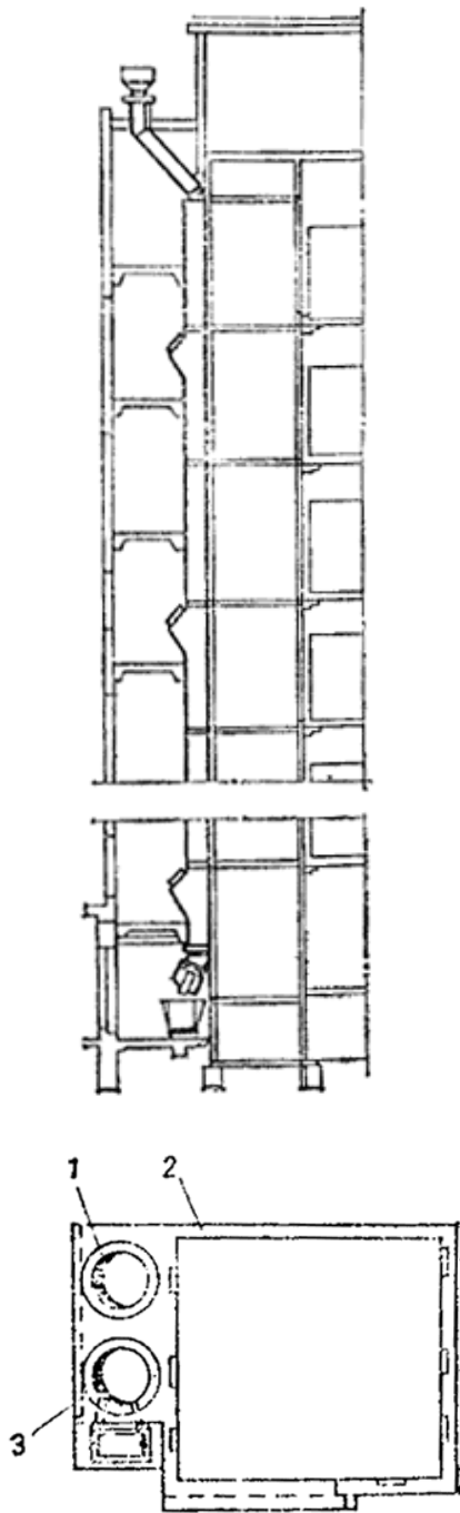
Рис. 15. Схема ствола мусоропровода, совмещенного с лифтовой шахтой
