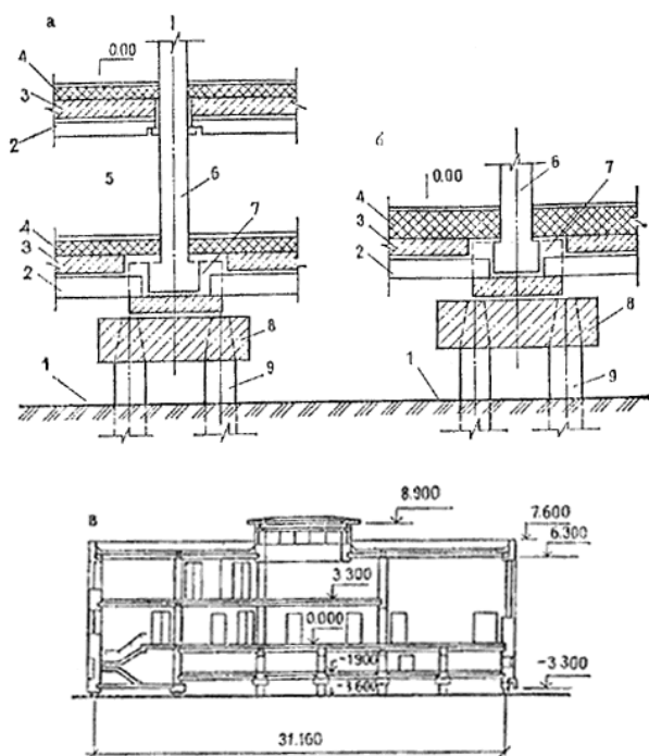
Рис. 1. Цокольно-фундаментная часть здания каркасной конструкции (1 принцип строительства)
