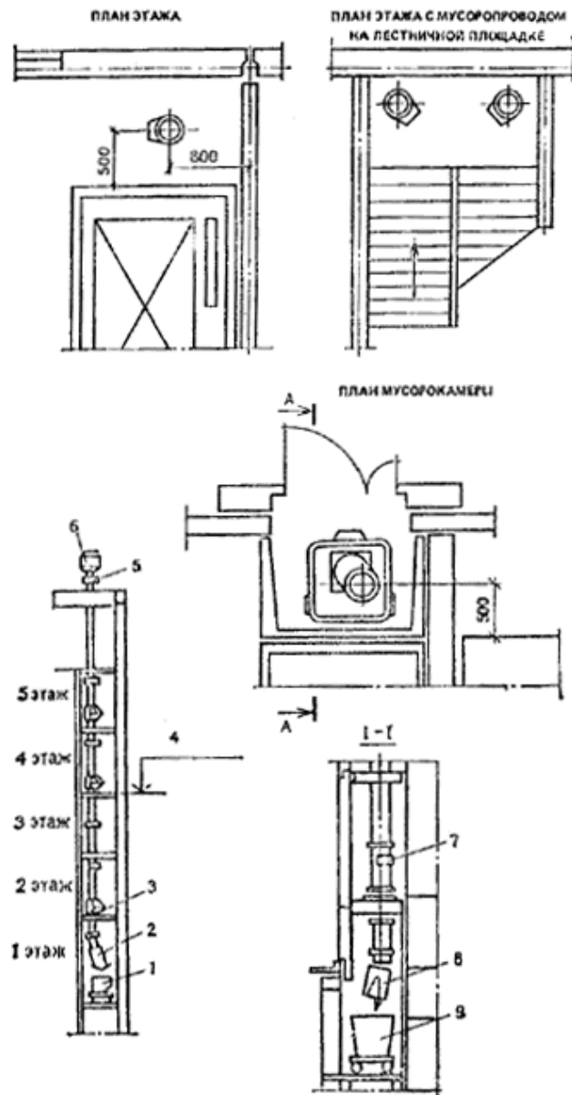
Рис. 13. Примерные схемы мусоропроводов
