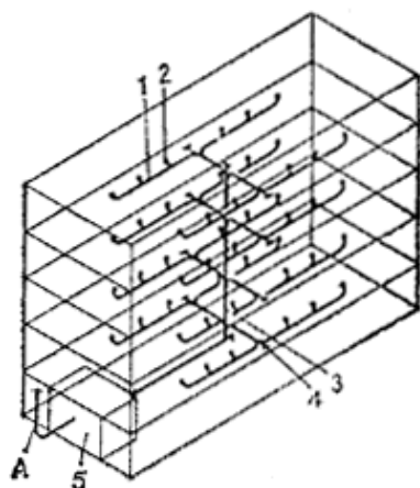
Рис. 12. Схема вакуумной централизованной пылеуборки с вертикальным магистральным пылепроводом
