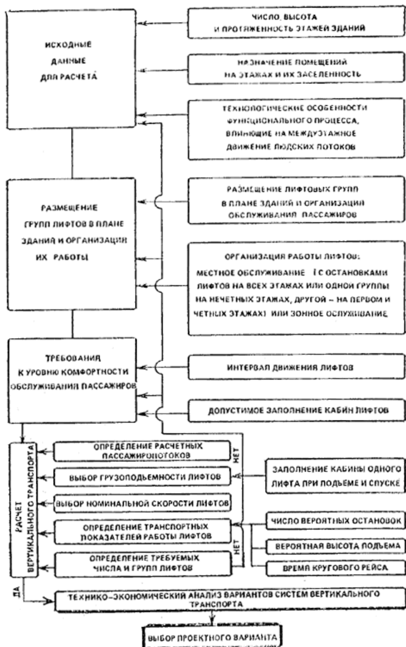
Блок-схема расчета вертикального транспорта
