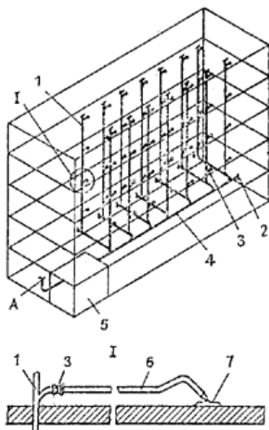
Рис. 11. Схема вакуумной централизованной пылеуборки с горизонтальным магистральным трубопроводом
