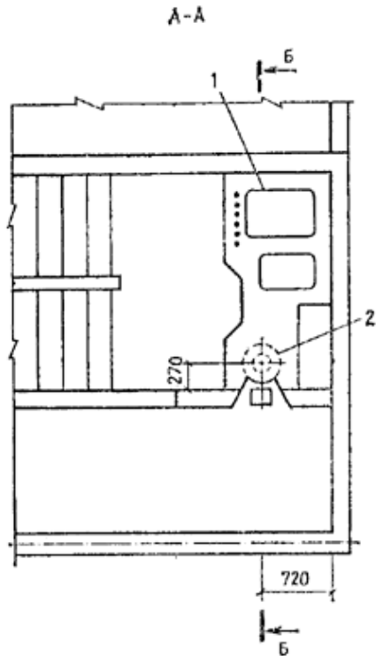
Рис. 16. Схема ствола мусоропровода, совмещенного с вентиляционным блоком
