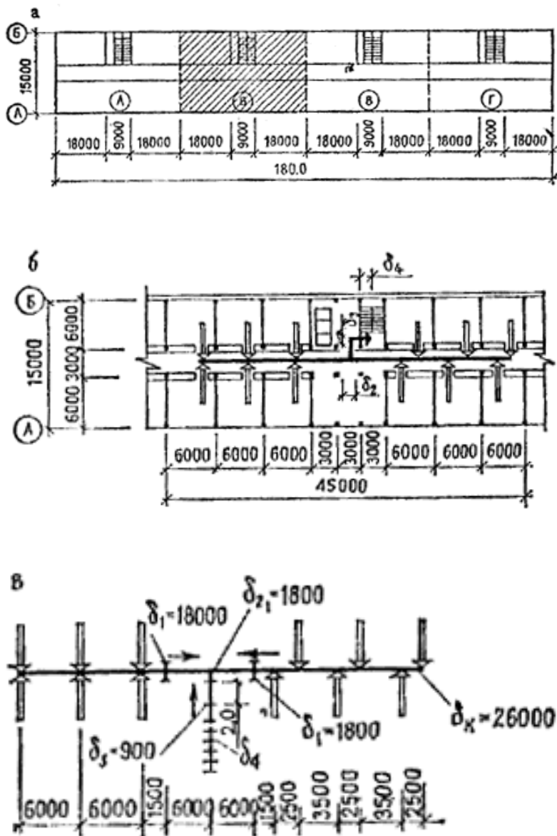
Схема плана типового этажа технического вуза
