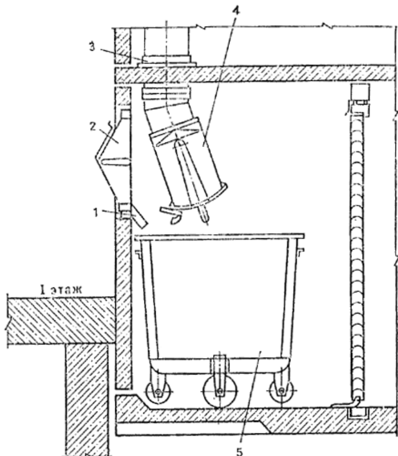
Рис. 14. Установка загрузочного клапана в стене мусоросборной камеры 1 — лоток; 2 — клапан загрузочный; 3 — опора ствола мусоропровода; 4 — направляющий патрубок с шибером; 5 — контейнер
