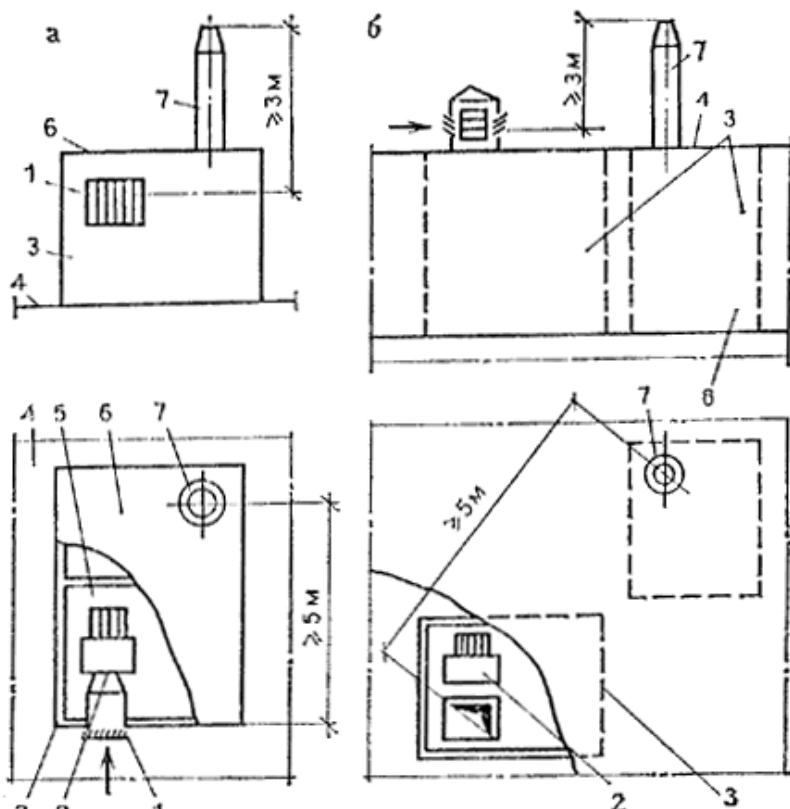
Рис. 28. Взаимное расположение отверстий воздухозабора и выброса дыма системы противодымной защиты зданий
