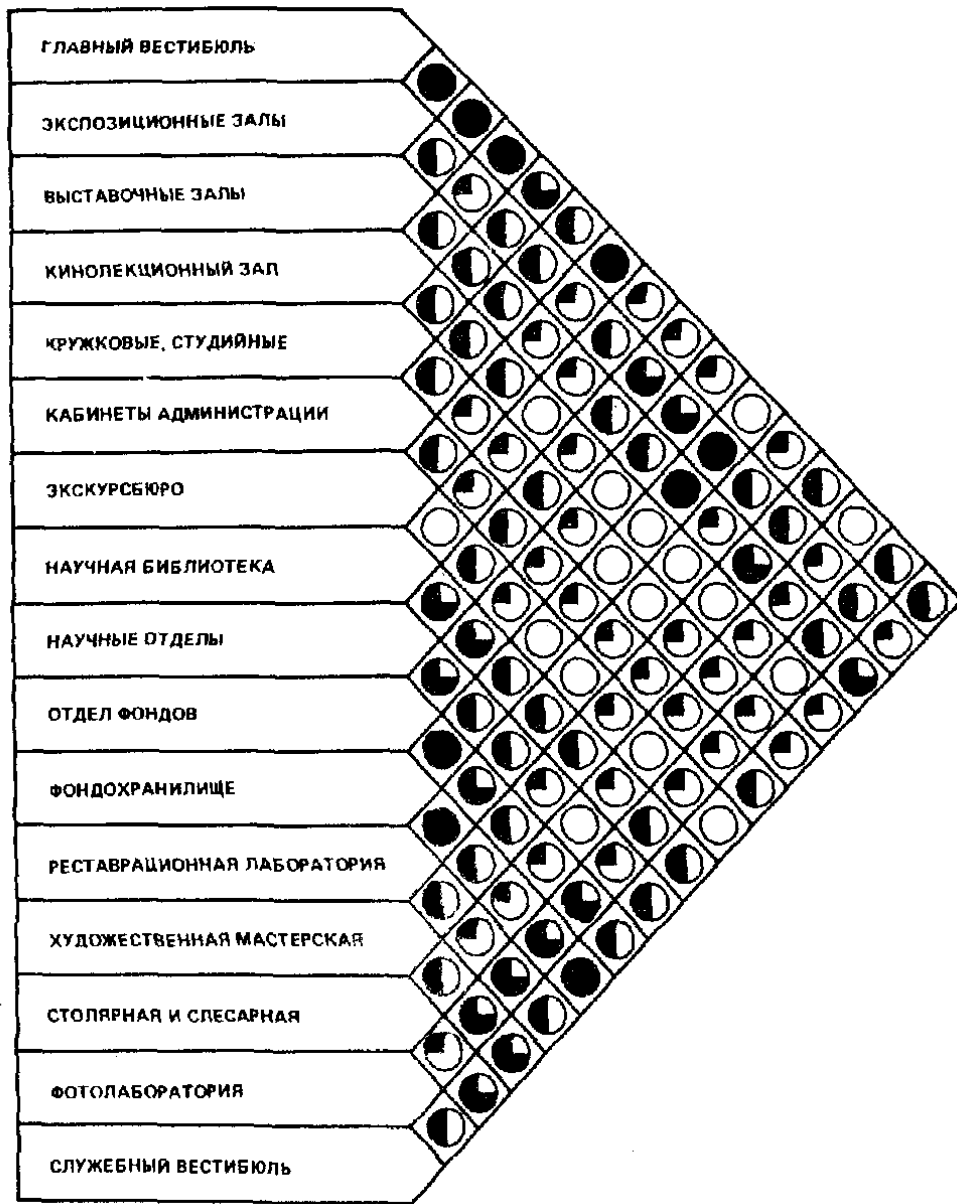
Рис. 2. Рекомендуемая степень взаимосвязи помещений
