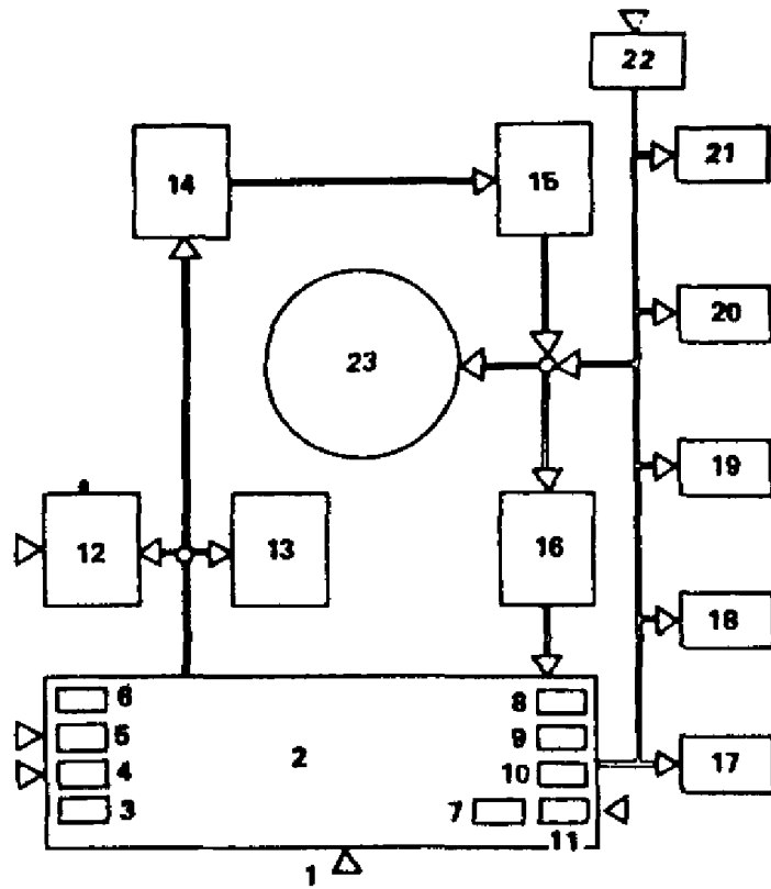
Рис. 16. Состав и взаимосвязь помещений панорамы
