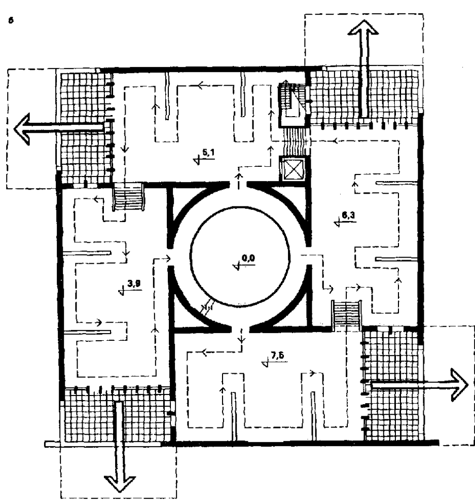
Рис. 12. Проект картинной галереи, обеспечивающей расширение здания по вертикали (а - разрез) и горизонтали (б - план в уровне экспозиции)
